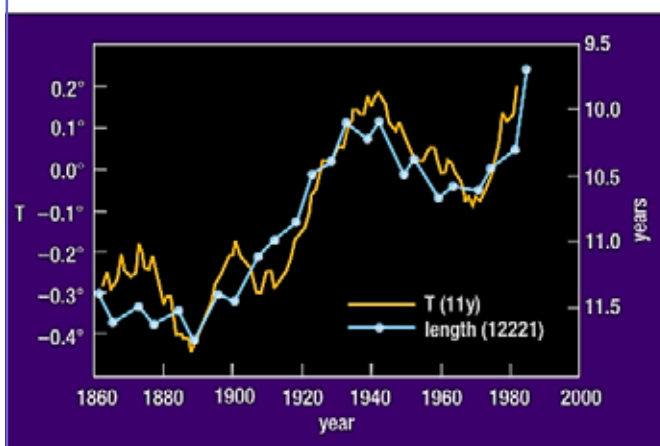
Sambandet mellan temperatur och solfläcksaktivitet
